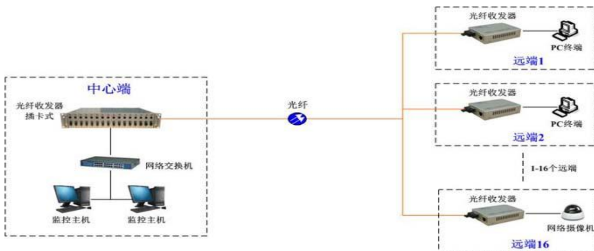
光纤点对多点组网
